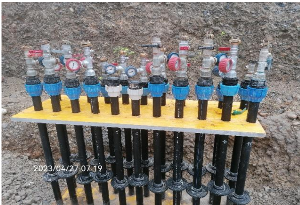
Drucküberwachung während der Aushubarbeiten
