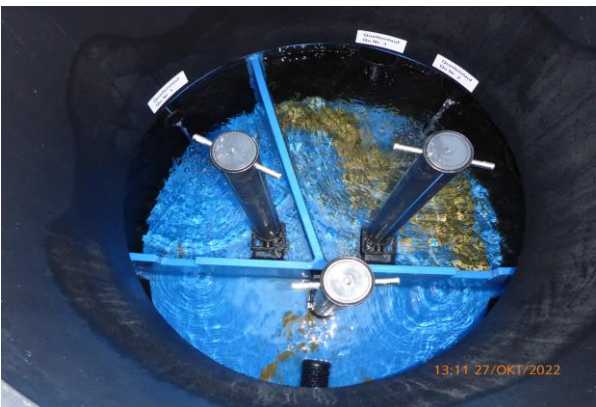
Sammelschächte sind der Wassermenge und Anzahl Quellfassungen angepasst
