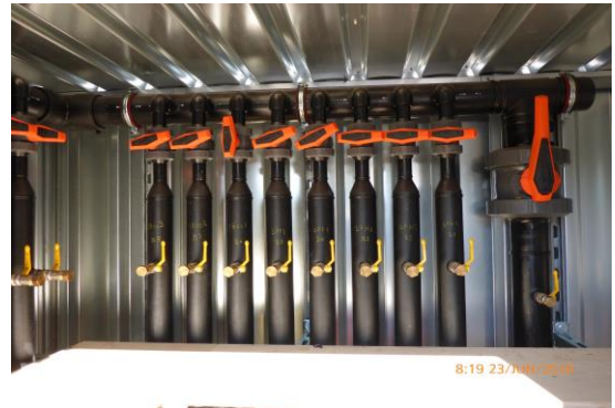
In der Zentrale werden alle Gasbrunnen zusammengefasst. Das Gas wird in den Brennofen abgeleitet.
