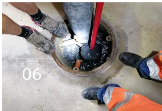
Reinigung der Gasbrunnen, Schächte und Verbindungsleitungen.
