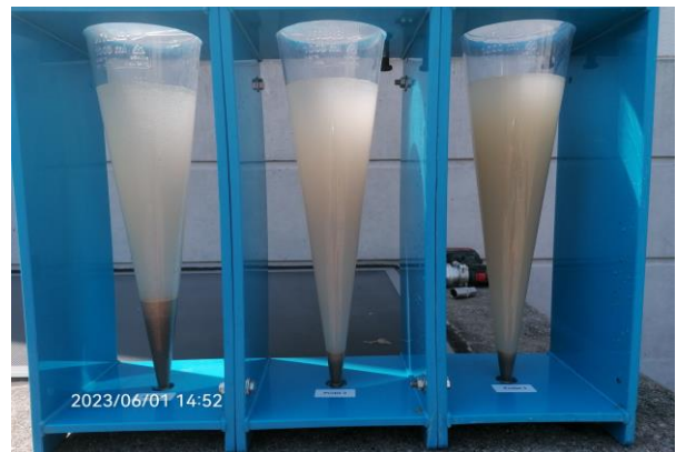
Prüfung der Sandfreiheit während der Brunnenreinigung
